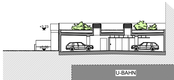
SCHNITT B
